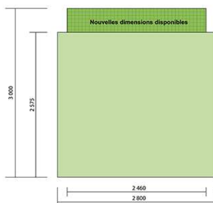
Bloc-porte 2 vantaux égaux
